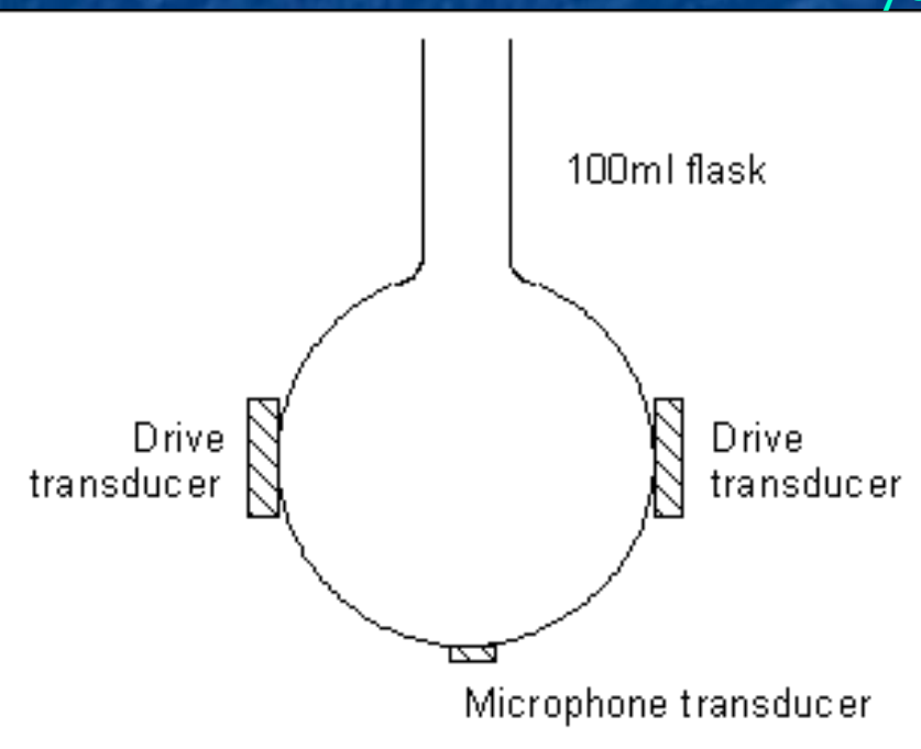
Схема установки
